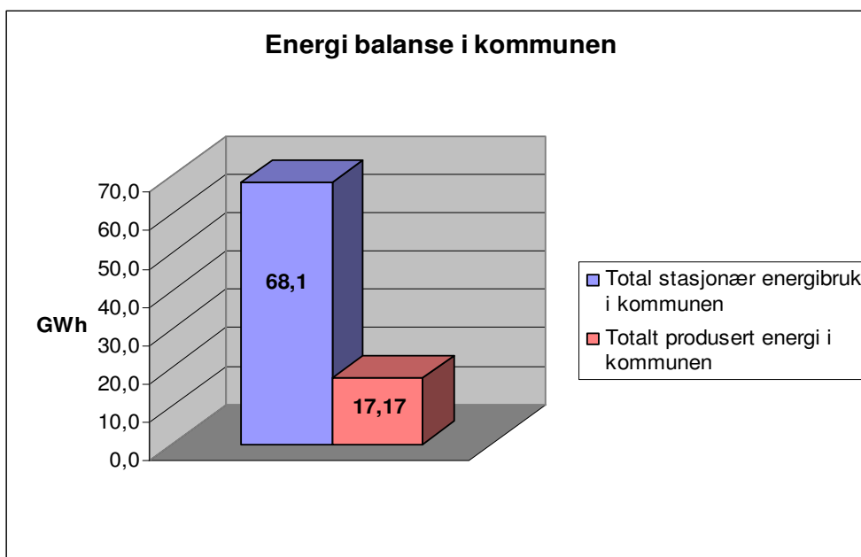
Fig. 1-2 Energibalansen i Overhalla i 2005.
