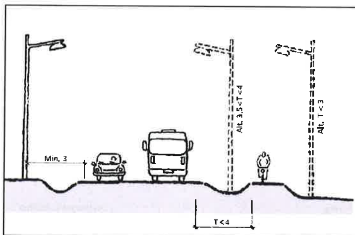
Figur 4-6 Plassering av master ift hovedveg og gang- og sykkelveg avhengig av trafikkløperens bredde (T). Kilde: Figur 4.8, håndbok V124, Statens vegvesen.
