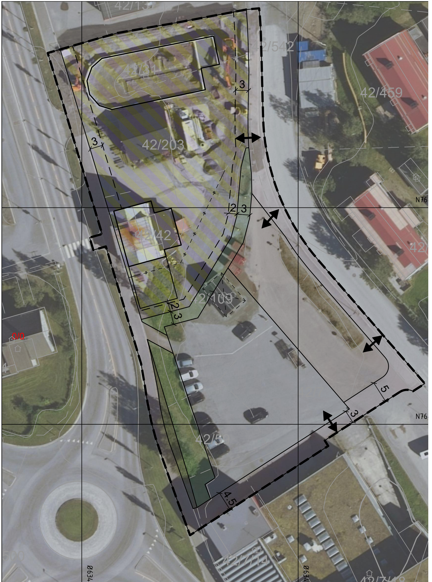
Illustrasjonsplan - Planforslag over ortofoto M=1:1000
