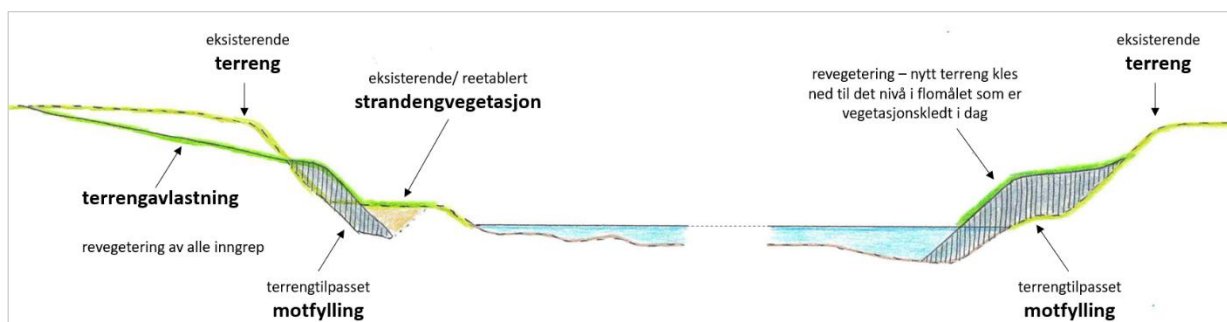
Figur 48: Prinsipp motfyllinger Tørrfjordelv – ikke målsatt
