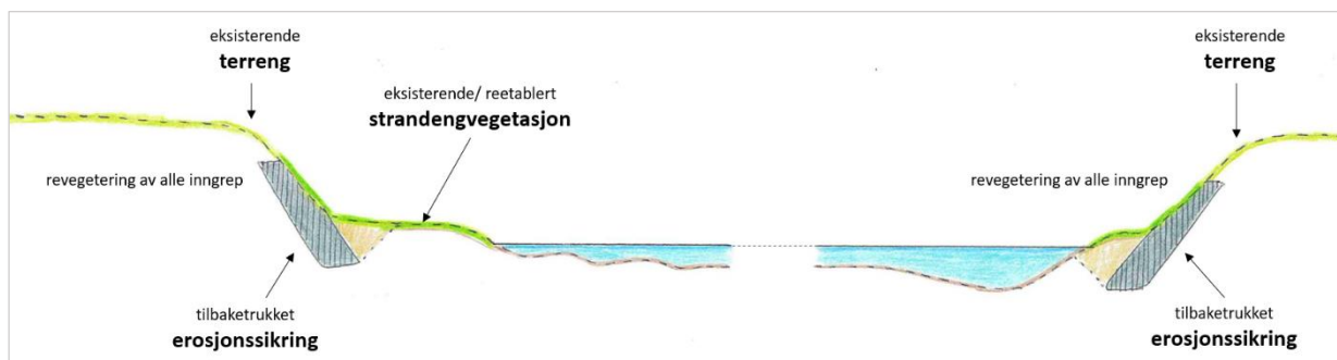
Figur 49: Prinsipp tilbaketrunket erosjonssikring Tørrfjordelv – ikke målsatt
