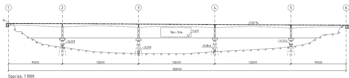
Figur 37: Profil Torkelseng bru
